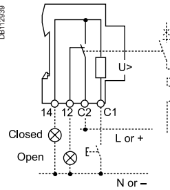
Wiring diagrams
