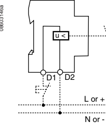
Wiring diagrams
