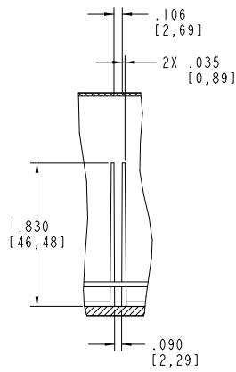
DETAIL C SCALE 1.500 TYP 24 PLACE
