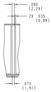
SCALE 2.000
