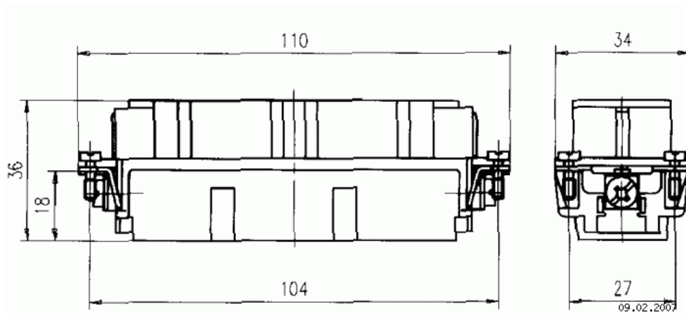
Maßzeichnung Dimensions in mm (Inch)
